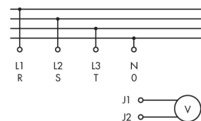
Kapcsolási rajz
