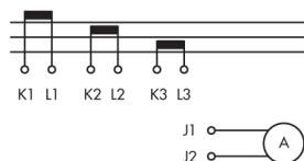
Kapcsolási rajz
