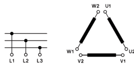
Kapcsolási rajz
