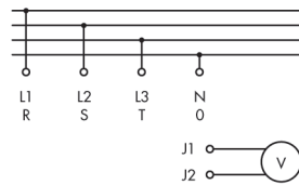
Kapcsolási rajz
